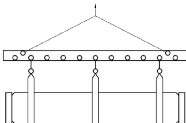
图 3 大口径石油工业用软管的搬运
